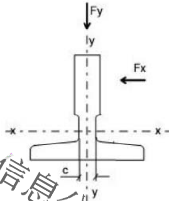
图 G1 导轨的坐标系
